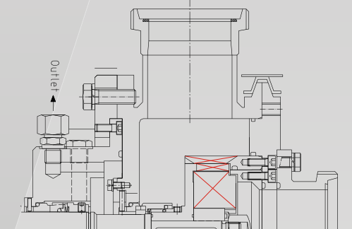
Combinaison Rotor / Stator 1 rotor denté/ 1 couronne - stator hélice de pompage
