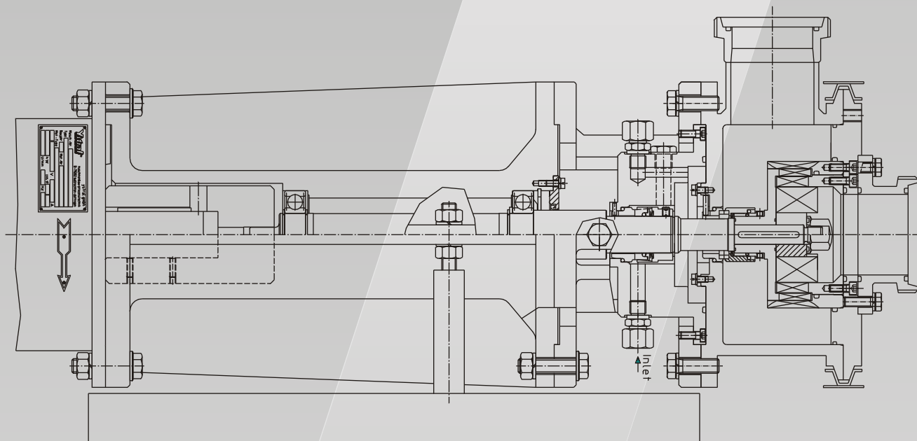
Combinaison Rotor / Stator 1 rotor denté/ 1 couronne - stator hélice de pompage
