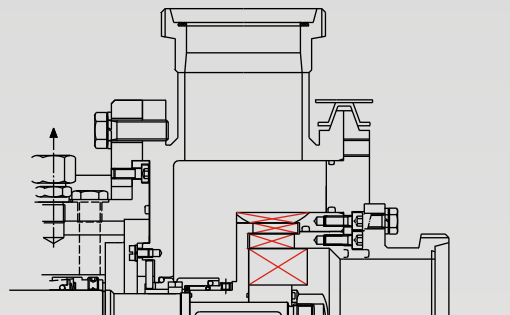
Combinaison Rotor / Stator 1 rotor denté / 2 couronnes - stator hélice de pompage
