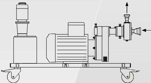
Z 132 monté sur châssis à roulettes avec pompe de recirculation pour lubrification des garnitures
