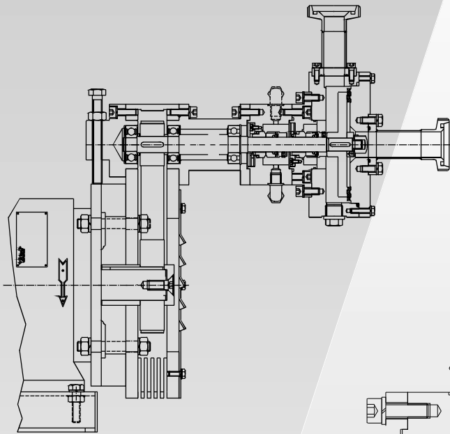
Z 132 avec entraînement par courroie
