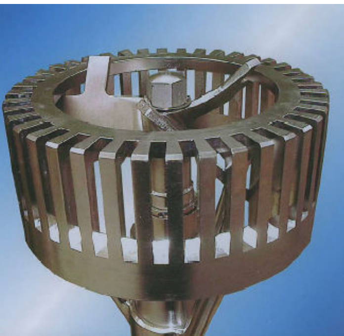
Rys. 1.: System rotorowostatorowy zawiera urządzenie szarżowe z pierścieniem tnącym. Głowica przypomina mieszadło strumieniowe, które w o wiele większym stopniu niż inne mieszadła przetwarza dostarczoną energię w pionowy strumień w zbiorniku.
